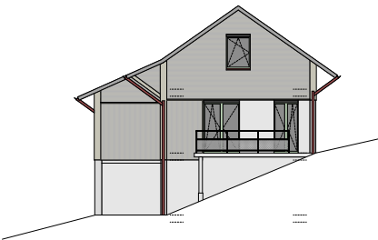
ANSICHT OST
